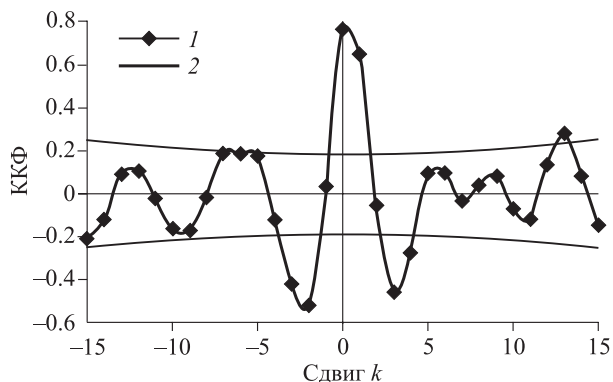
Рис. 3. Кросс-корреляционная функция временных рядов температуры в мае 2014 г. по данным метеостанций Енисейска и Богучан.
