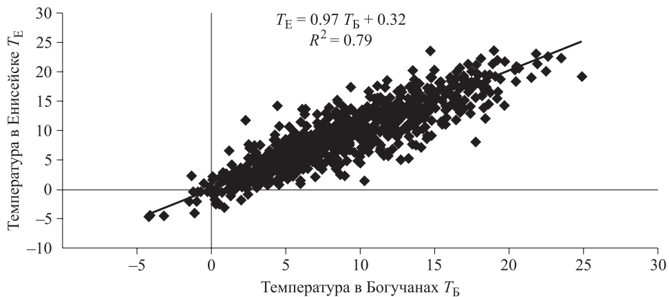
Рис. 1. Связь между температурами (на 12 ч дня) по данным метеостанций Енисейска ( T_E ) и Богучан ( T_B ) в течение дней мая 1988–2019 гг.
