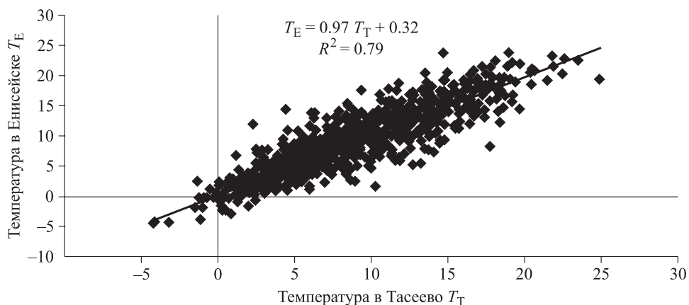
Рис. 2. Связь между температурами (на 12 ч дня) по данным метеостанций Енисейска и Тасеево в течение дней мая 1988 – 2019 гг.
